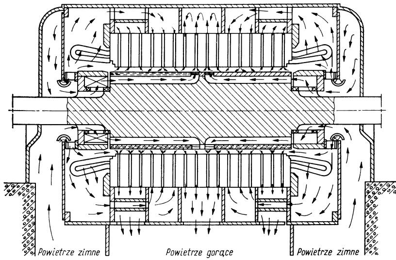
Schemat trójstrugowej wentylacji powietrznej pośredniej
