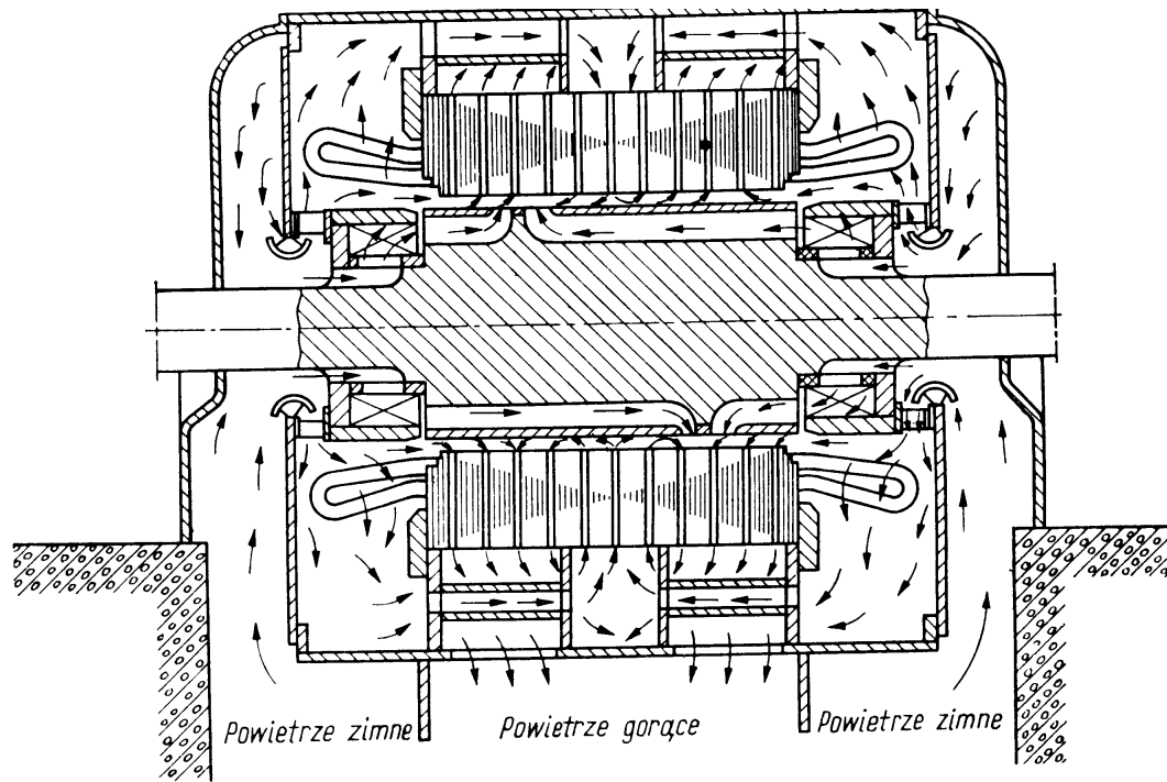
Schemat dwustrugowej wentylacji powietrznej pośredniej
