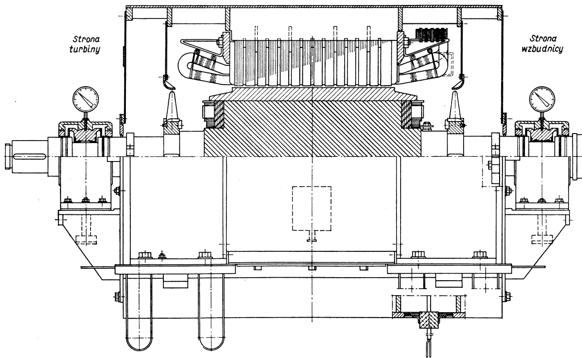
Przekrój podłużny czterobiegunowego turbogenerators dużej mocy
