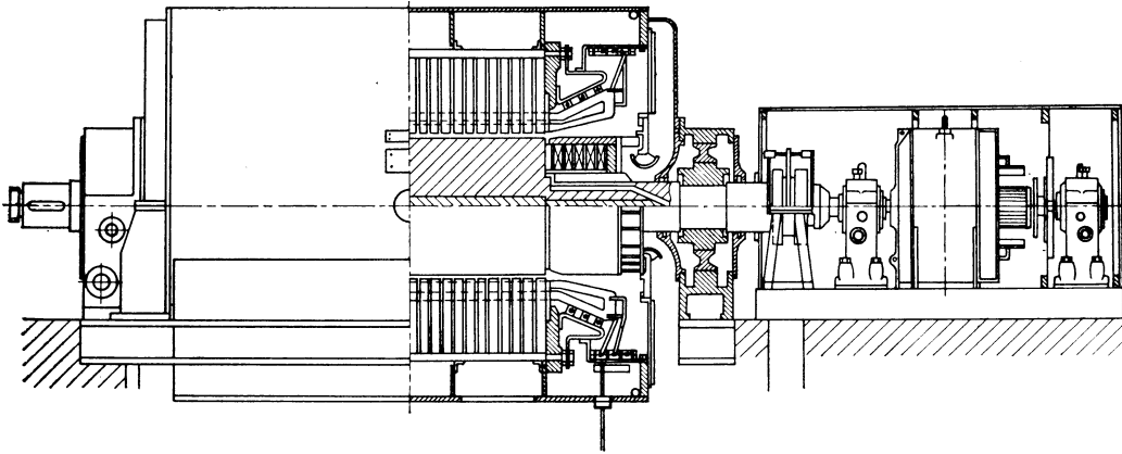
Ogólny widok turbogenerators z chłodzeniem pośrednim powietrznym
