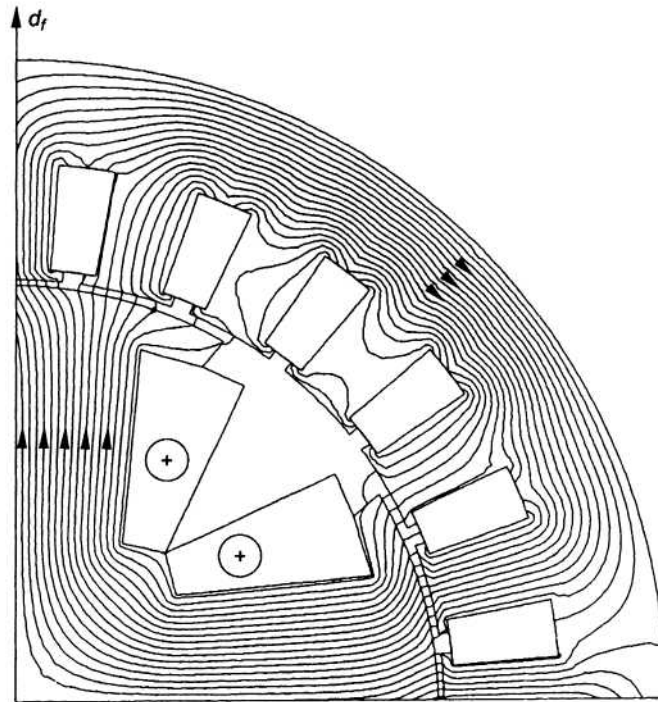
Rozkład chwilowy pola magnetycznego w maszynie synchronicznej wzbudzanego przepływem prądu w uzwojeniu skupionym na biegunach wirnika (magneśnicy)
