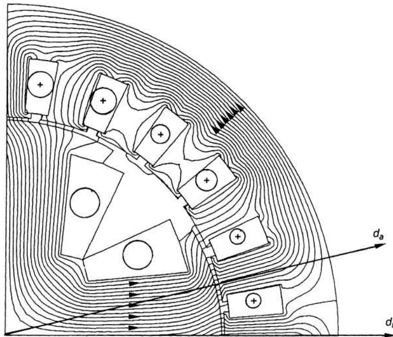
Rozkład chwilowy pola magnetycznego w maszynie synchronicznej wzbudzanego przepływem prądu w uzwojeniach twornika na stojanie
